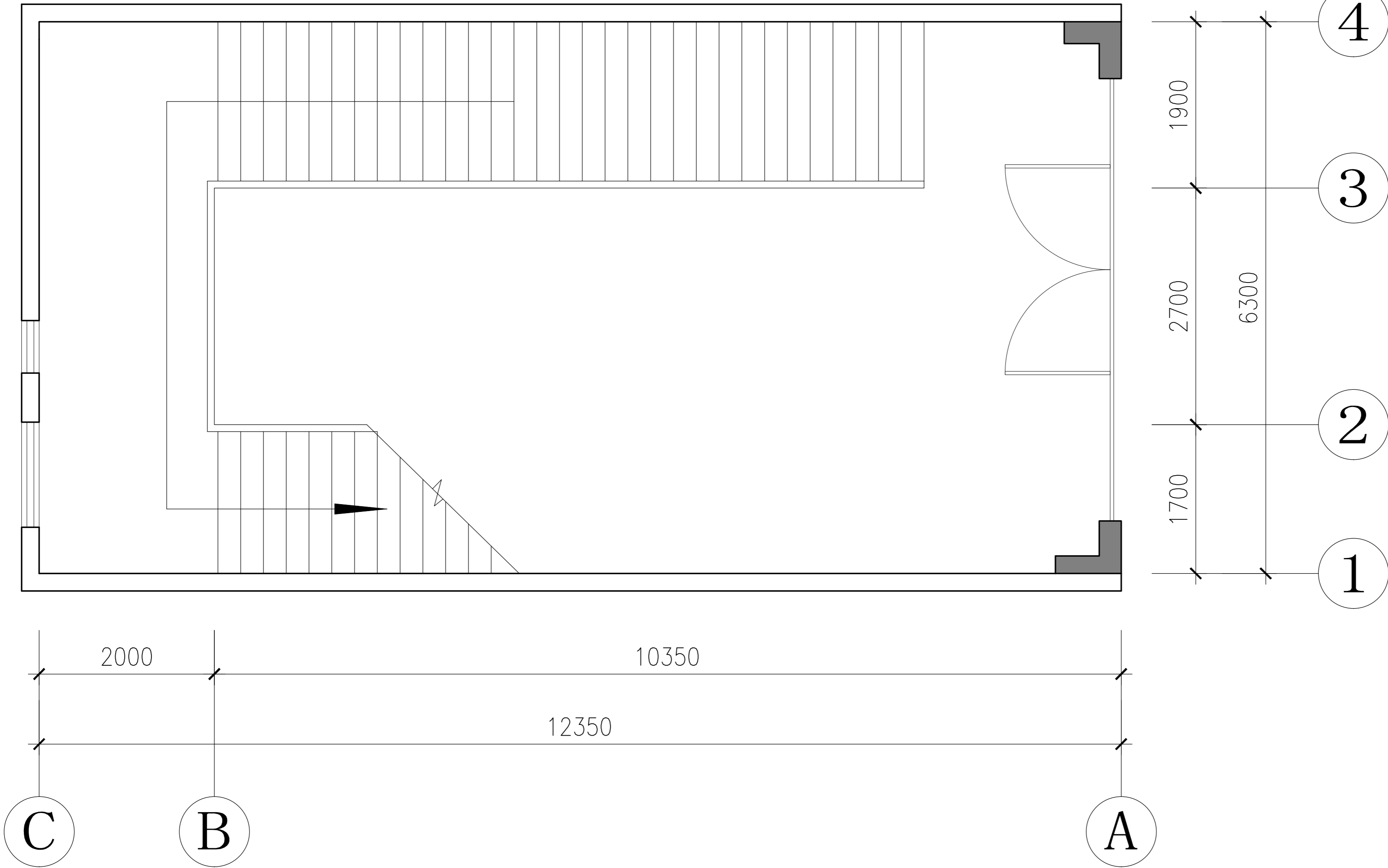
一层原始结构图 SC : 1:100
